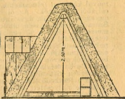
21. II. keresztmetszet.
